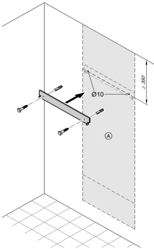
(A) Монтажный шаблон
